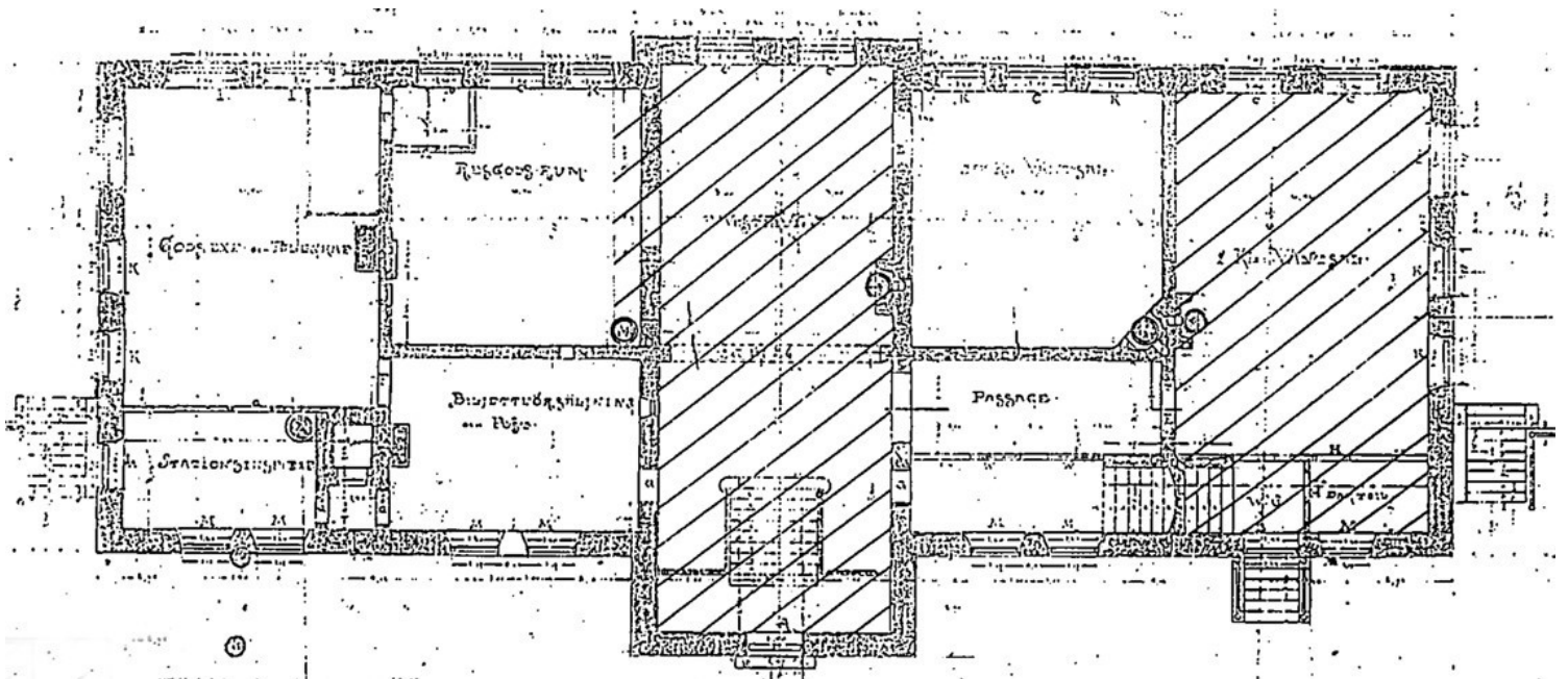
Planlösning. Interiören på bottenvåningen med dess stenmurar. Streckade områden fick inte röras
